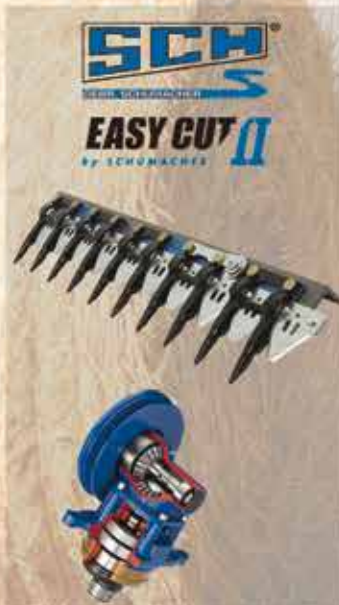
Sistemas de corte para cosechadoras con rodillos guía. Grupos de sierra horizontales, verticales. Levantamieses.
