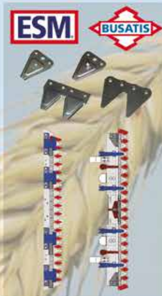
Cortes accionamiento doble BUSATIS. Estándar y Bidux. Cortes accionamiento simple ESM. Secciones y Componentes.
